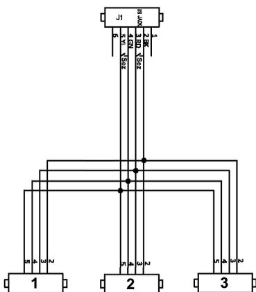
Schema elettrico (schematic diagram)
